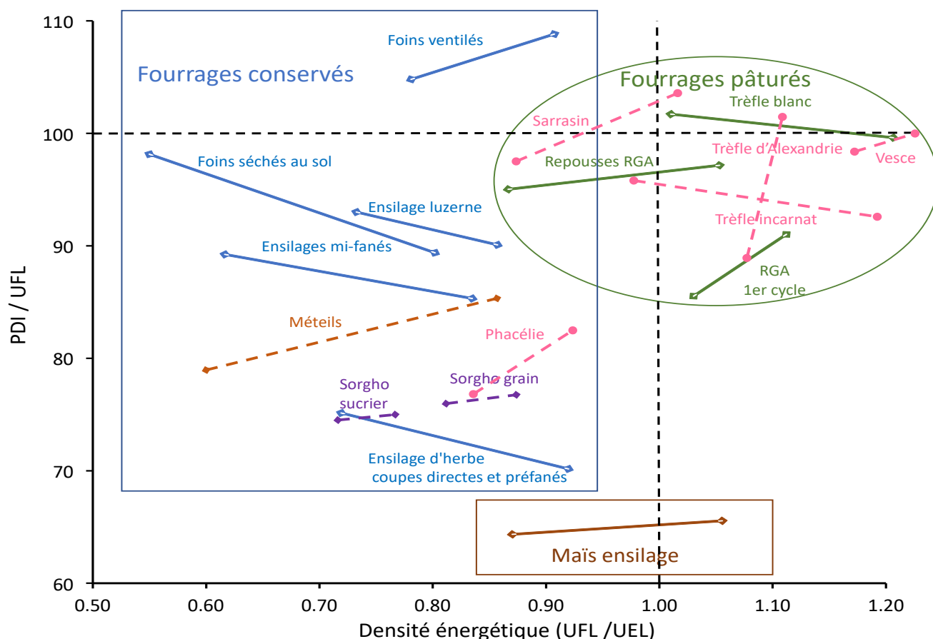
Figure 1. Relations entre la densité énergétique des fourrages et leur concentration en protéines digestibles par unité fourragère. Les traits pleins correspondent aux fourrages des tables INRA (INRA, 2018) et représentent la plage de variation renseignée selon le stade d'exploitation du fourrage. Les traits pointillés représentent des catégories de fourrages non renseignées dans les tables INRA : en rose, des espèces fourragères utilisées en dérobées estivales (Maxin et al., 2020) ; en violet des valeurs pour les ensilages de sorgho estimées à partir des données de Brunschwig et al., (2008) et de Chauveau et Uijtewaal (2020) ; en marron les données sur les méteils estimées à partir de Legendre et al., (2019).
