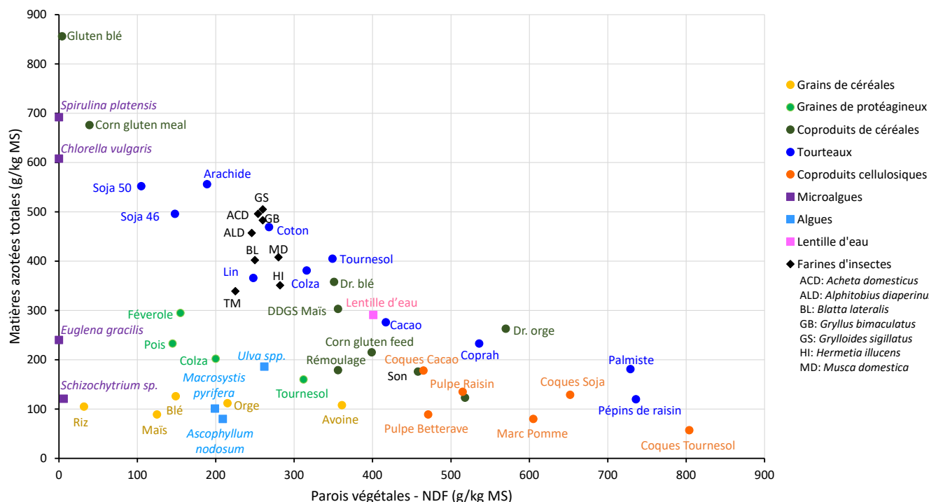
Figure 2. Teneurs moyennes en protéines (MAT) et en parois végétales (NDF) pour les principaux groupes de matières premières actuellement utilisées ou potentiellement utilisables en alimentation des ruminants.
